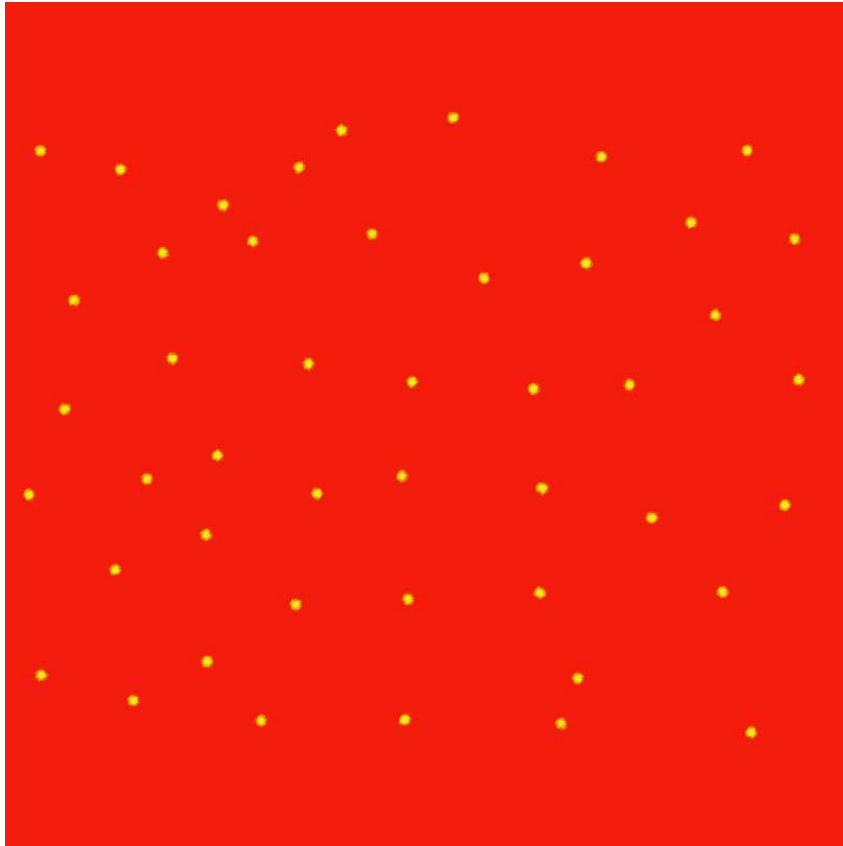
UNIFORME
