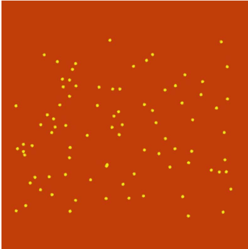
ALEATÓRIO
