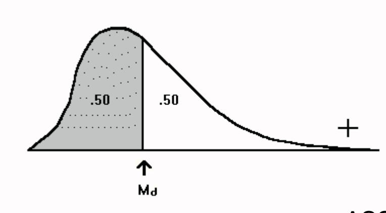
ASSIMETRIA
